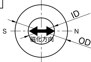
上面図
